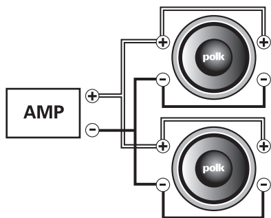
Figure 9 With coils and speakers wired in parallel, two dual 4 Ohms speakers will present a 1 Ohm load. (Not recommended unless amplifier is rated for 1 Ohm operation.) Deux haut-parleurs, à bobines 4 Ohms jumelées configurées en parallèle, câblés en parallèle constituent une charge de 1 Ohm. (Non recommandé à moins que l'amplificateur soit capable de soutenir une charge de 1 Ohm.) Con las bobinas y los altavoces en paralelo, 2 altavoces de dos bobinas y 4 Ohms presentan una carga de 1 Ohm. (Se recomienda no utilizar este cableado a menos que el amplificador tenga una clasificación nominal para funcionar con 1 Ohm.)
